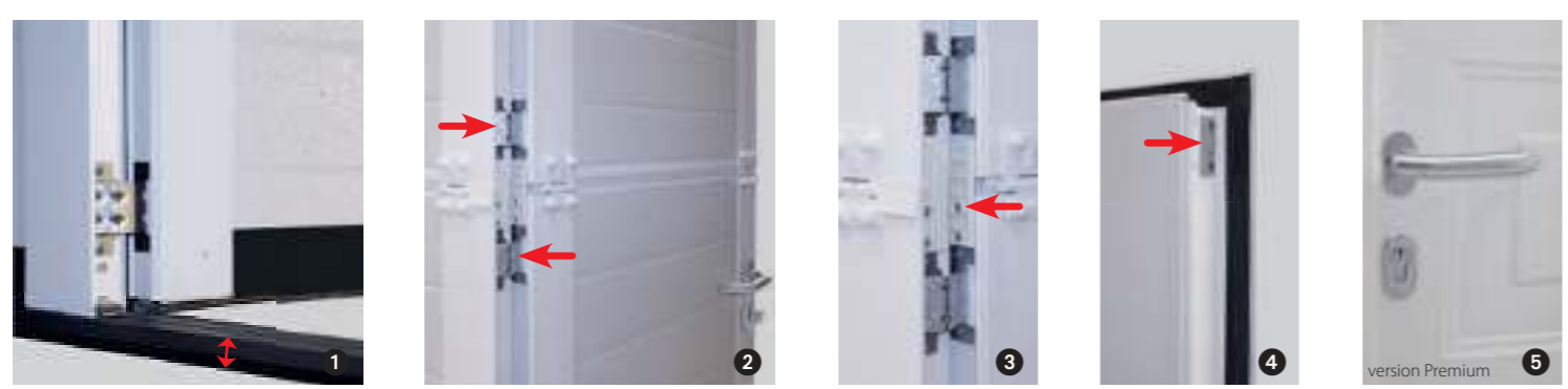
Porte sectionnelle Iso 45 à portillon, version Premium, design sans nervures, finition lisse. Options: hublots Réf. 1, gris 7016 sablé et automatisme.
